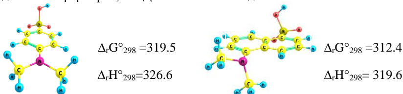
Рис. Структуры 4-ДМАБСК и ДК ( \Delta_r G^\circ_{298} и \Delta_r H^\circ_{298} в ккал/моль)
