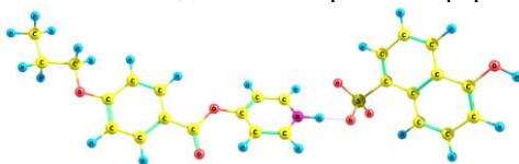
Рис. Структура комплекса ГНСК···ПЭ в различных растворителях
