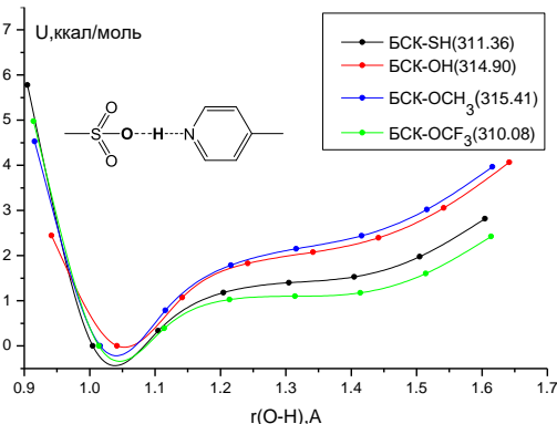
Рис. Потенциальная функция переноса протона в комплексах и величины \Delta_r G_{298}^0 газофазного депротонирования кислот, ккал/моль
