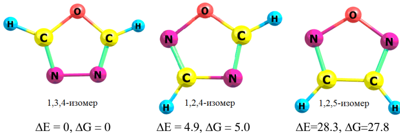
Рис. Структуры 1,2,4-, 1,3,4- и 1,2,5-оксадиазола ( \Delta E и \Delta G в ккал/моль)
