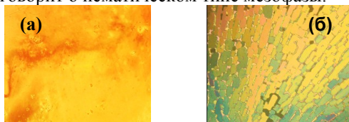
Рис. Мраморная текстура нематической мезофазы Н-комплекса 4-ЭОКК+АП зарегистрированная в режиме нагревания (а); мозаичная текстура Н-комплекса 4-МОКК+АП , зарегистрированная в режиме нагревания (б)
