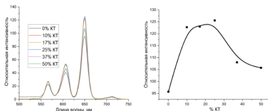
Рис. Усиление люминесценции комплекса самария в композите с квантовыми точками
